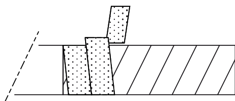
5. Tørk vekk eventuelt støv fra spirokanalen og REC Flex Combi. Fest teip over sømmen. Begynn 50 mm før og avslutt 50 mm etter SBF-klemmen.
