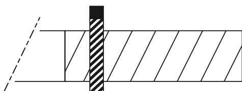
3. Fest REC Flex Combi med en SBF-slangeklemme.
